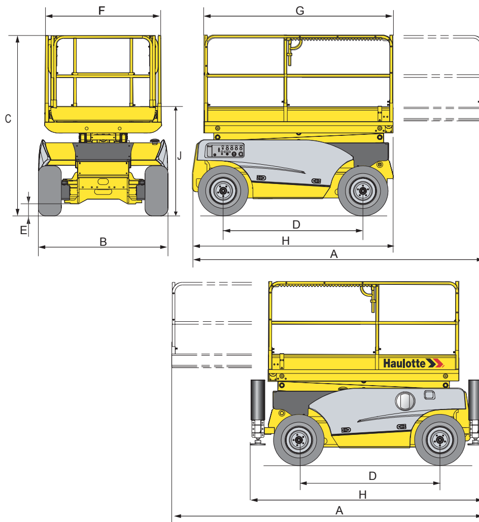
Спецификация габаритных размеров
